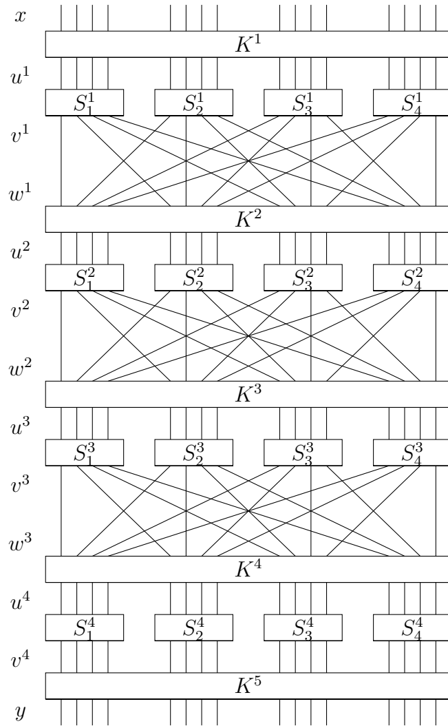
Abbildung 4.1: Ein Substitutions-Permutations-Netzwerk.
