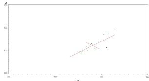
Länge und Breite von Venusmuscheln mit Hauptkomponenten
