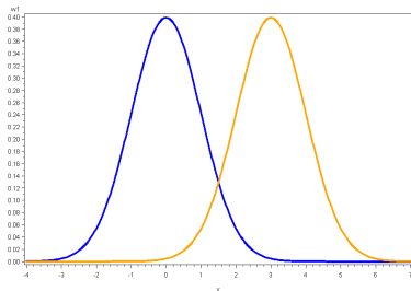
Dichtefunktion verschiedener Normalverteilungen
