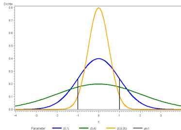
Dichtefunktion verschiedener Normalverteilungen
