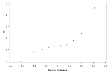
TTEST-Daten
