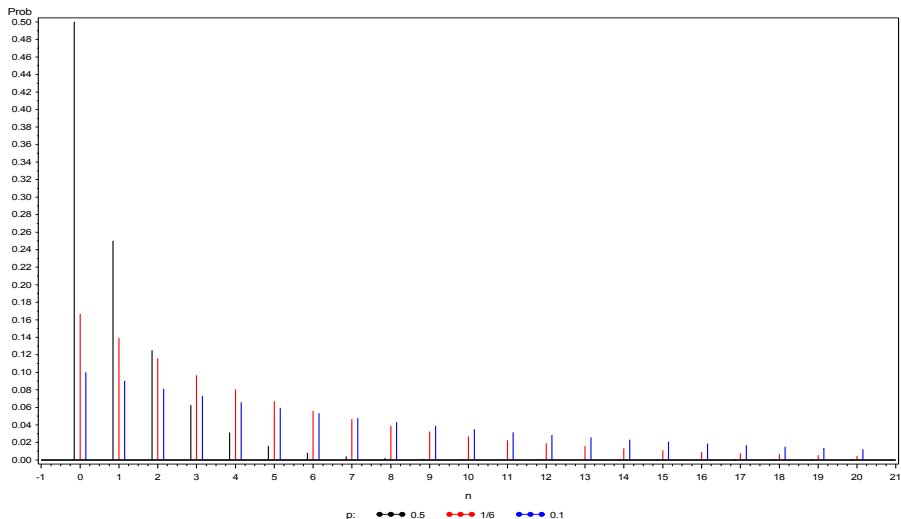
Geometrische Wahrscheinlichkeiten mit p=0.5, 1/6, 0.1
