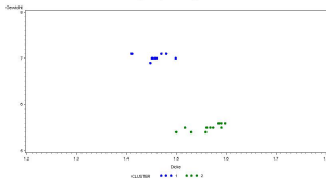
Byzantinische Münzen Single-Linkage Cluster Analyse
